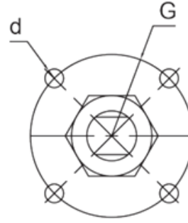
AKTÜATÖR BAĞLANTISI
