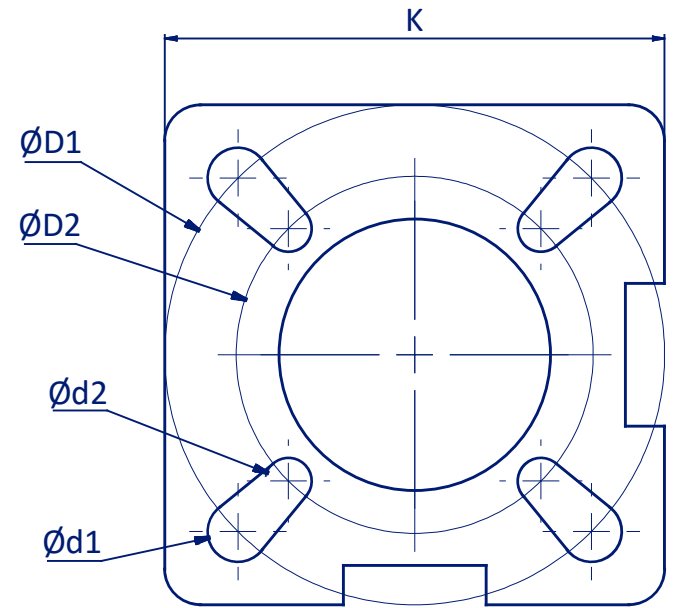
ISO5211 FLANGE DIMENSIONS
